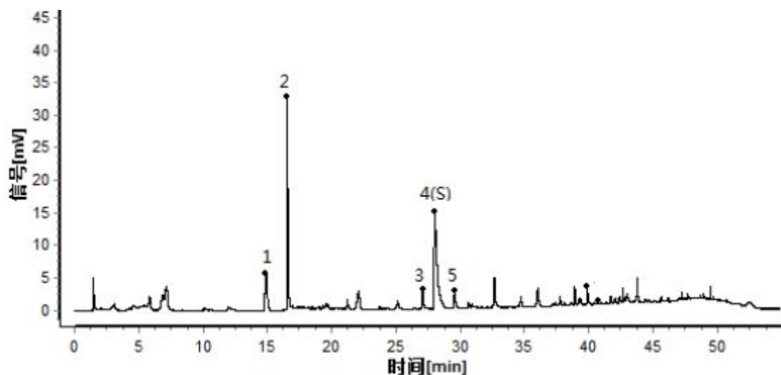
峰 4(S)：芥子碱硫氰酸盐 芥子（白芥）配方颗粒对照特征图谱 色谱柱：CORTECS T3；2.1mm×150mm，1.6μm
