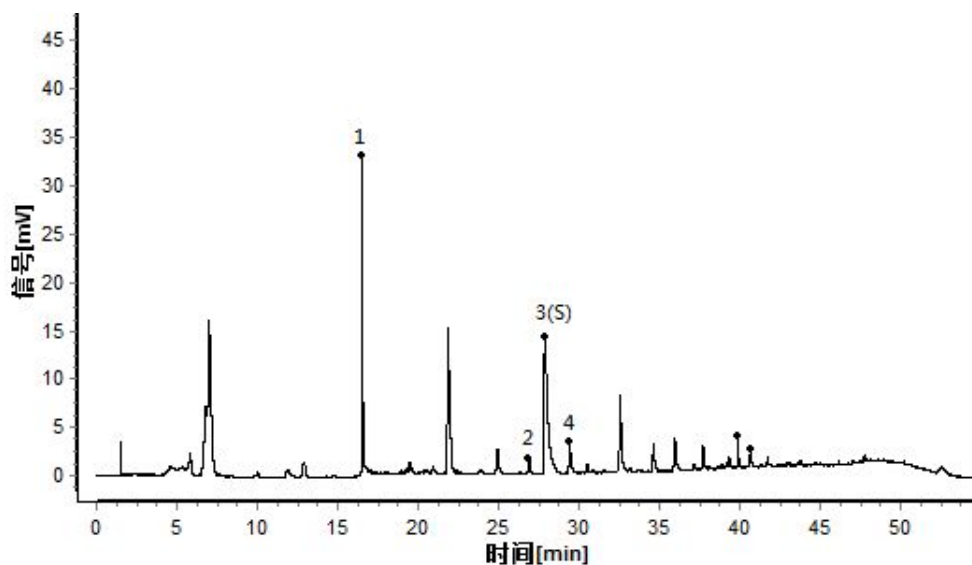
峰 3(S)：芥子碱硫氰酸盐 炒芥子（白芥）配方颗粒对照特征图谱 色谱柱：CORTECS T3；2.1mm×150mm，1.6μm
